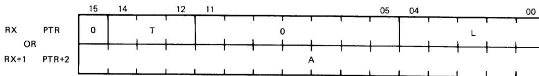
Figure 14-5 Decimal String Descriptor
