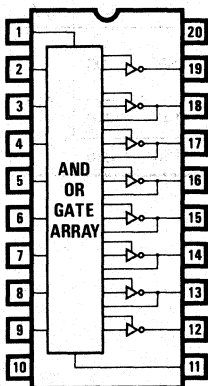
PAL16L8
